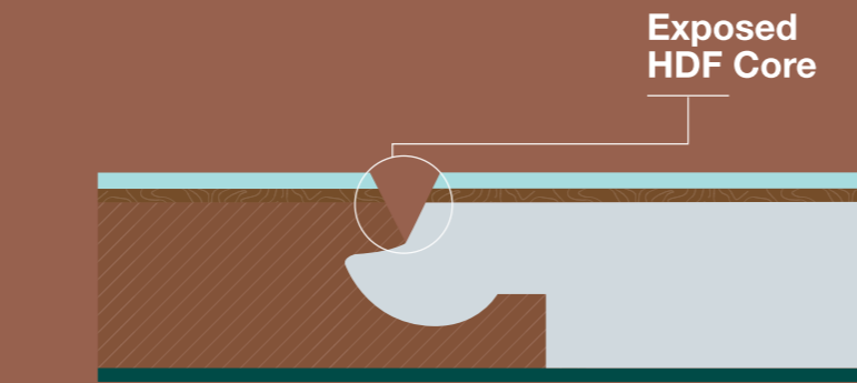
V-GROOVE (FIG.3)
